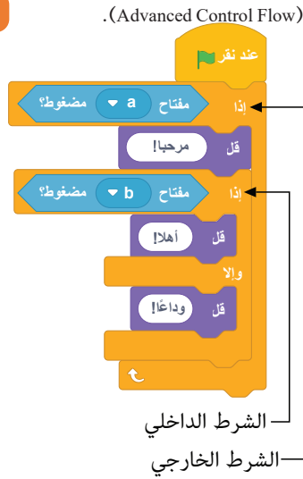
الشكل (2-2): مثال على كتلة برمجية باستخدام التحكم المتقدم.
